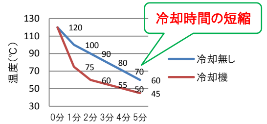
冷却温度比較(室温約35℃)
